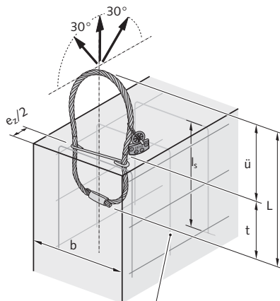
Fig. 2: Montage transversal
