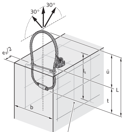
Abb. 2: Einbau quer
