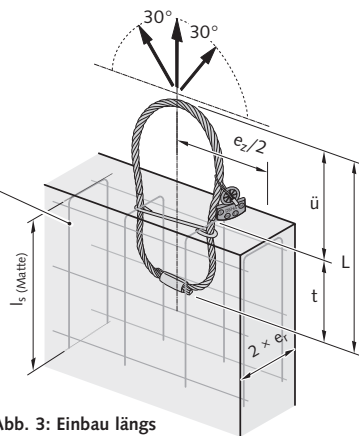
Abb. 3: Einbau längs
