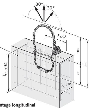
Fig. 3: Montage longitudinal
