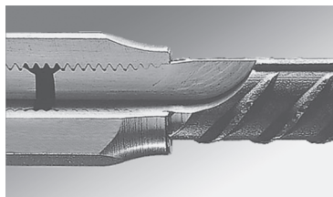
Przekrój skręconego połączenia
