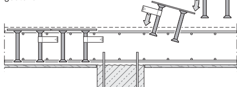
Fig. 3: De ponswapeningselementen worden van boven door de reeds aanwezige bovenwapening gestoken
