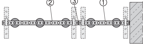
Figure 3: Inserte los elementos HDB desde arriba a través del refuerzo superior
