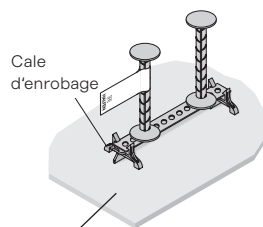
Coffrage en bois ou en acier
