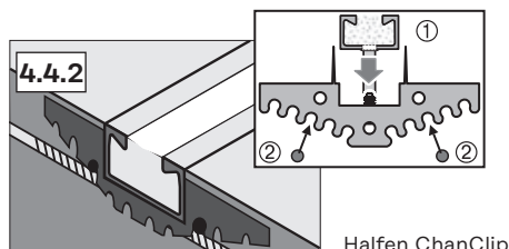
Halfen ChanClip
