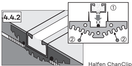
Halfen ChanClip
