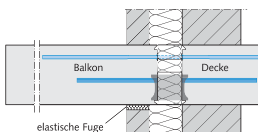
Zweischaliges Mauerwerk bei deckengleichem Balkon
