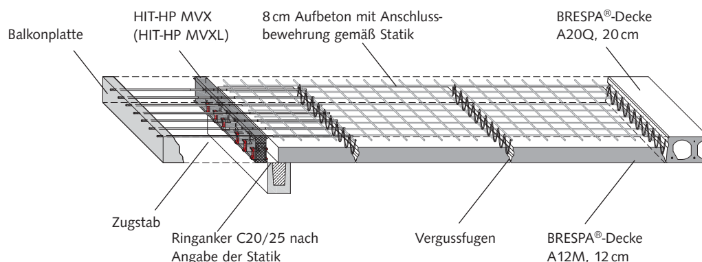
Abb: Balkonanbindung durch HALFEN HIT-Elemente und Aufbeton an BRESPA® Massivdecken
