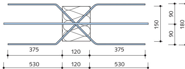
Draufsicht HIT-SP HT4
