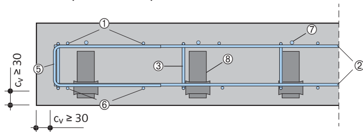
Schnitt B-B, Beispiel HIT-MVX
