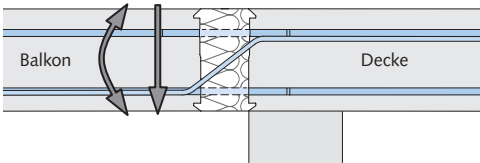
HIT-HP DVL – High Performance mit 80 mm Dämmstärke
