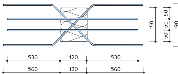
Draufsicht HIT-SP HT5
