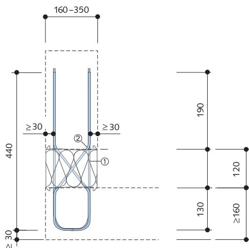
Querschnitt: HIT-SP AT1
