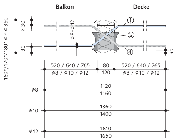
Abbildung: Typ HIT-SP ZVX-0404...-08 gerade Ausführung; Querkraftstäbe \phi 8 , \phi 10 , \phi 12 mm (als Sonderkonstruktion auch in \phi 6 mm lieferbar)
