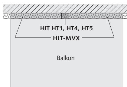
Anwendung: Frei auskragender Balkon
