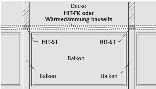
Anwendung: Wärmegedämmter Anschluss von Konsolen
