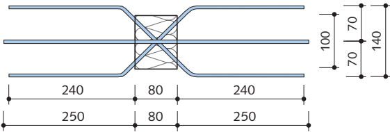
Draufsicht HIT-HP HT3
