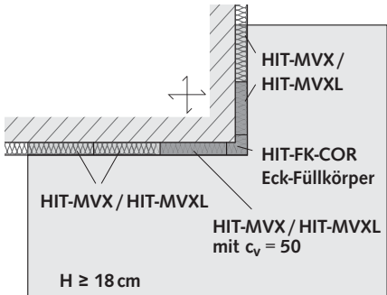
Anwendungsbeispiel: Außenecke
