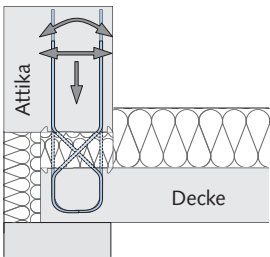
Anwendung: Geschossdecke mit Attika
