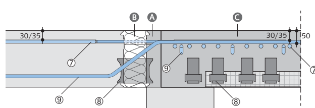
Darstellung der HIT-Elemente im Eck-Bereich mit Elementdecke
