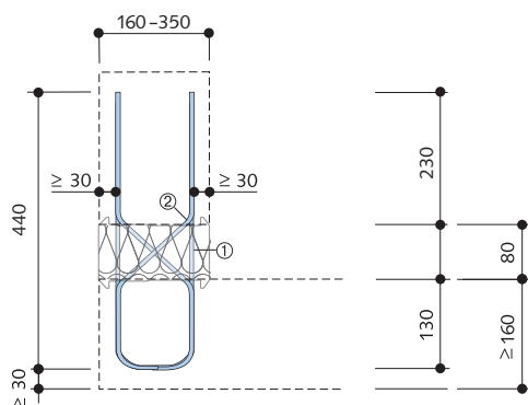
Querschnitt: HIT-SP AT1
