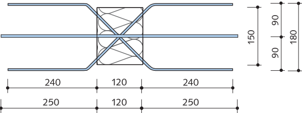
Draufsicht HIT-SP HT3
