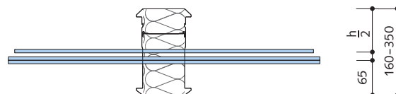
Draufsicht HIT-HP HT5
