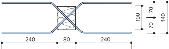
Draufsicht HIT-HP HT1
