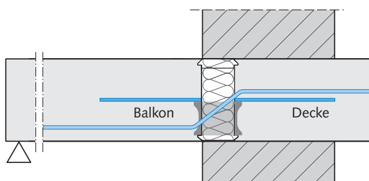
Einschaliges Mauerwerk bei deckengleichem Balkon
