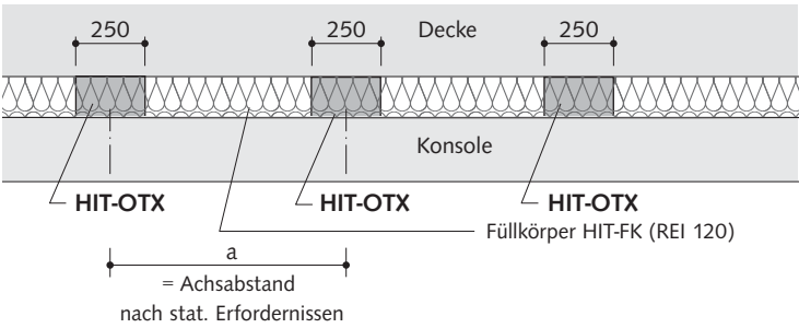
Draufsicht: Decke mit angeschlossener Konsole
