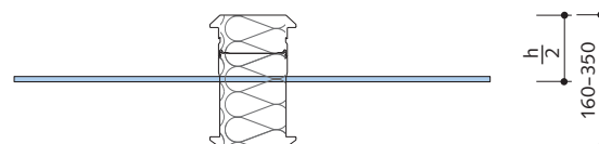
Draufsicht HIT-HP HT2
