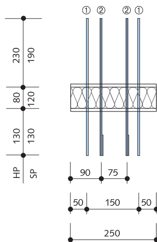
Draufsicht: HIT-HP/SP AT1 – Stababstände
