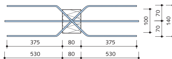
Draufsicht HIT-SP HT4
