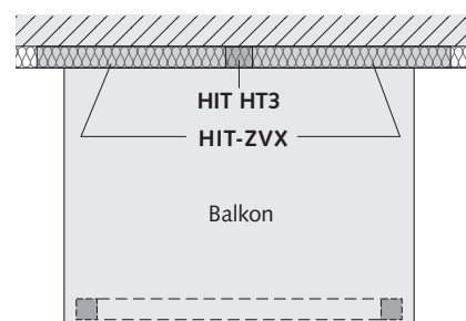
Anwendung: Balkon mit Stützenauflagerung
