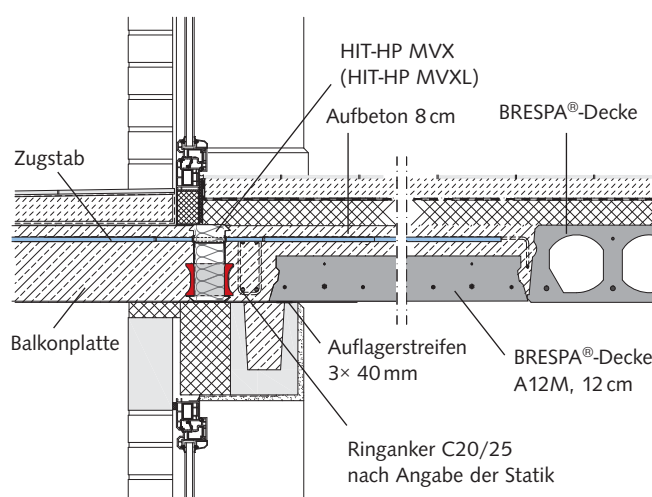
Abb: Balkonanschlüsse an BRESPA®-Massivdecke (Beispiel)
