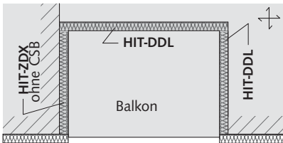
Anwendung: Durchgehende Platten
