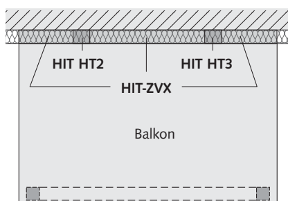
Anwendung: Balkon mit Stützenauflagerung
