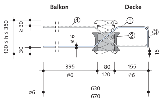
Abbildung: Typ HIT-SP ZVX-0404...-06 gebogene Ausführung; Querkraftstäbe \phi 6 mm (als Sonderkonstruktion auch in \phi 8 mm lieferbar)
