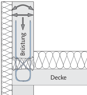
Anwendung: Geschossdecke mit einer hohen Attika bzw. Brüstung
