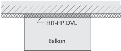
Anwendung: Frei auskragender Balkon
