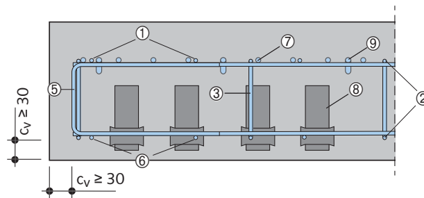
Schnitt B-B, Beispiel HIT-MVXL
