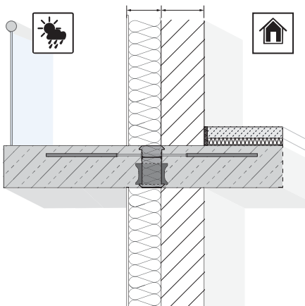
Abb. 1: Querschnitt durch eine Balkonplatte mit HALFEN HIT- Element, angeschlossen an einer Innendecke.
