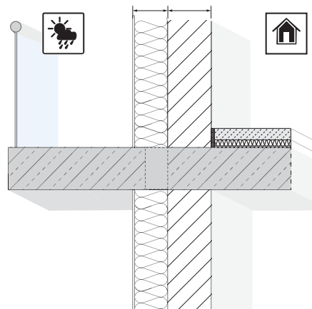
Abb. 2: Querschnitt durch eine Balkonplatte mit homogenem Ersatzkörper, angeschlossen an einer Innendecke.
