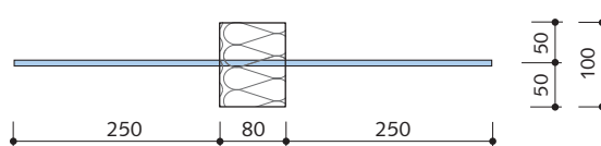
Draufsicht HIT-HP HT2
