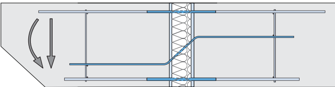
HIT-HP ST – High Performance mit 80 mm Dämmstärke HIT-SP ST – Superior Performance mit 120 mm Dämmstärke
