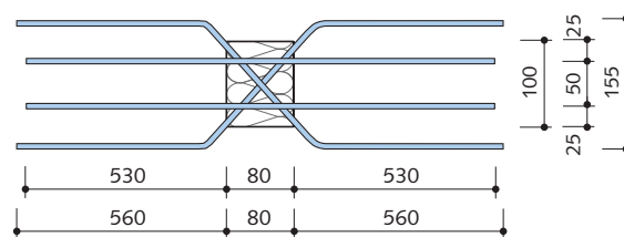
Draufsicht HIT-SP HT5
