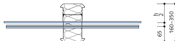
Draufsicht HIT-HP HT4
