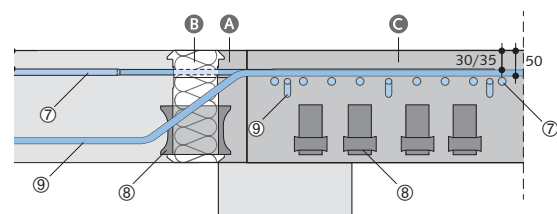
Darstellung der HIT-Elemente im Eck-Bereich
