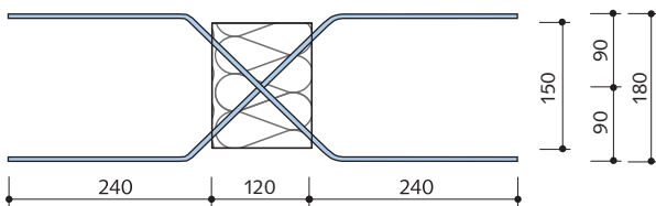
Draufsicht HIT-SP HT1
