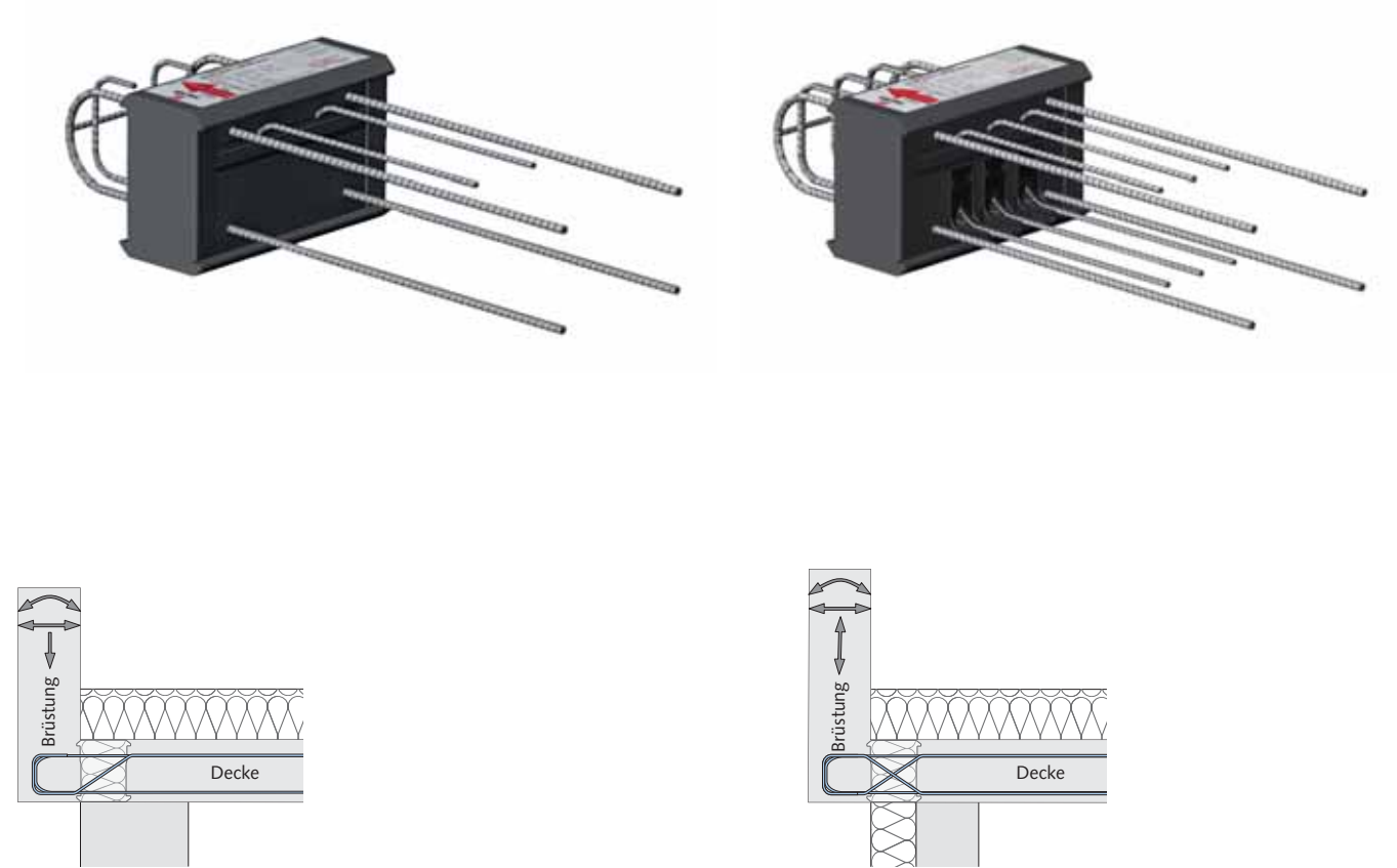
Querschnitt HIT-SP FT1: Geschossdecke mit einer vorgesetzten Brüstung und wärmedämmendem Mauerwerk
