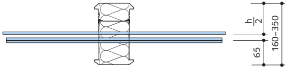
Draufsicht HIT-HP HT3
