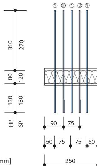
HIT-HP/SP AT2 – Stababstände
