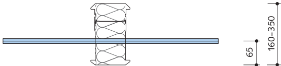
Draufsicht HIT-HP HT1
