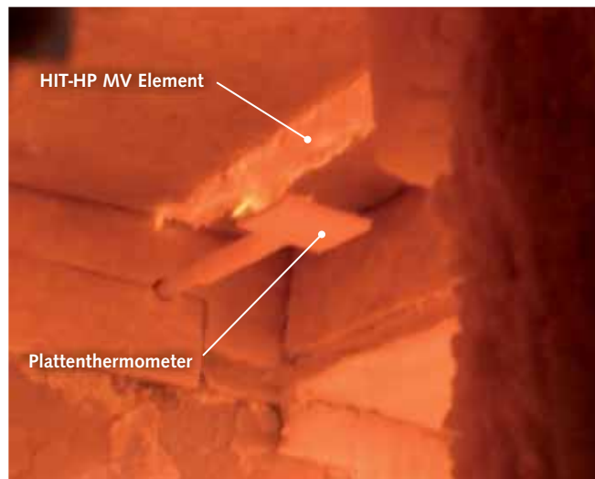
Sicht in den Brandraum während der Versuchsdurchführung HIT-HP MV nach 120 Min. Brandbeanspruchung
