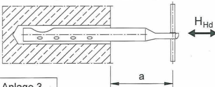
Anordnung in der Horizontalfuge
