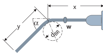
BG, 1x gebogen
