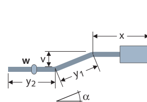
SG, gekröpft ③
