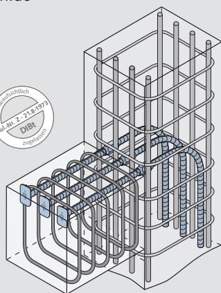
HSC Konsole kombiniert mit HALFEN HBS-05 Schraubanschluss
