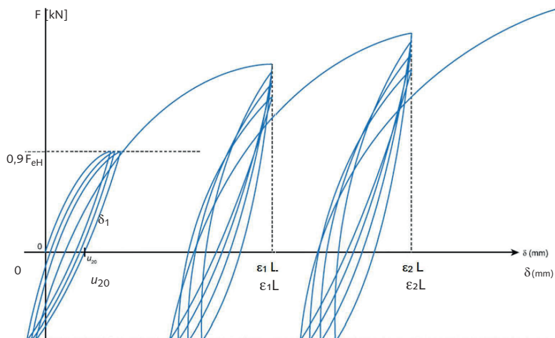
Diagramm: Lauf einer Versuchsreihe mit HBS-05-Seismic unter alternierender Zug-Druck-Belastung gemäß ISO 15835:2018.
