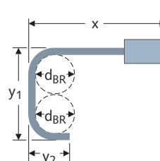
SG, 2x gebogen ③
