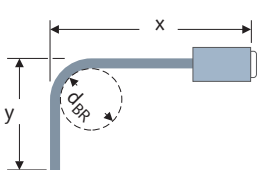
SG, 1x gebogen 90°
