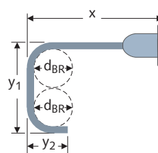
BG, 2x gebogen ③
