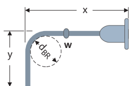
BG, 1x gebogen 90°
