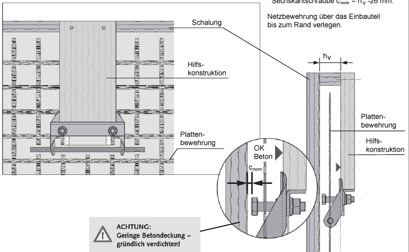
A2 Hilfskonstruktion an Schalung befestigen. Planmäßige Betondeckung unter Sechskantschraube c_{\text{nom}} = h_v - 26 \text{ mm} .
