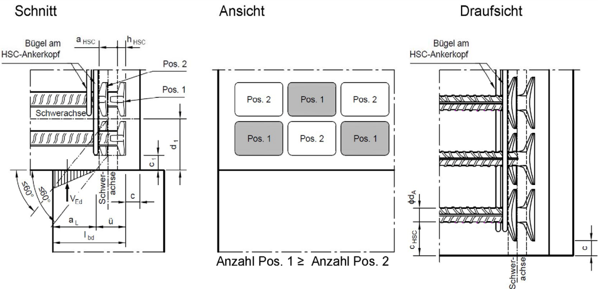
Abbildung 12: Anordnung zweilagig gestaffelter HSC-Anker mit dreiecksförmiger Lagerpressung, Beispiel
